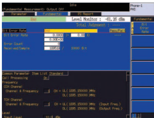
BER (8PSK)
